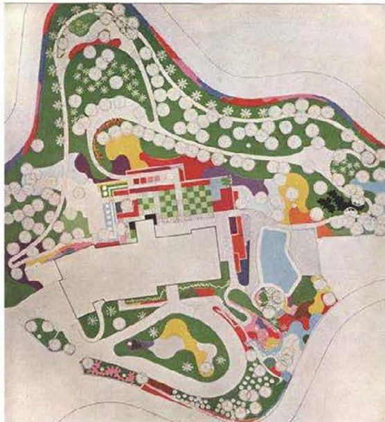
Figura 53. Plano del jardín de Palácios a color realizado por Burle Marx y los arquitectos asociados. Fuente: Revista Zedue, N° 6 (1968).
